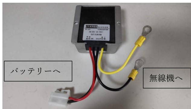
DCDC コンバータ (IN:9~13V OUT:13.8V18A)
